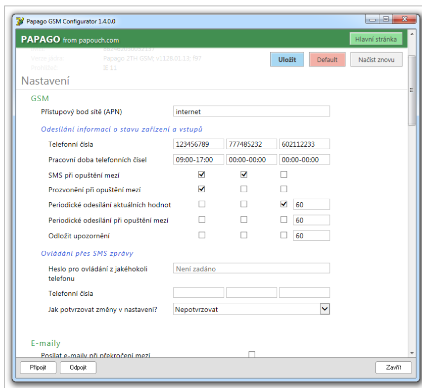
obr. 3 - Konfigurace Papaga
