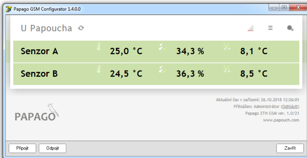
obr. 2 - Tři veličiny z teplotně-vlhkostního senzoru připojeného ke konektoru A na Papago 2TH
